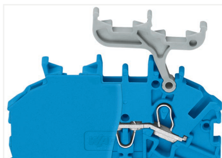
ダブルデッキマーカーキャリアは、角度を変え、ジャンパの着脱や結線作業が容易です
