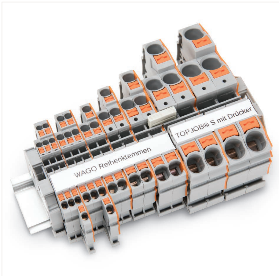
可とうより線 / より線： ドライバでボタンを押し、電線を入れます 電線を押さえたままドライバを離せば結線されます ※プッシュイン接続できない細い単線およびフェール 圧着線もボタン操作で結線可能です
