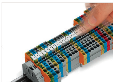
WMB 連続マーカ使用例 マークスロットにスナップインで取り付けできます
