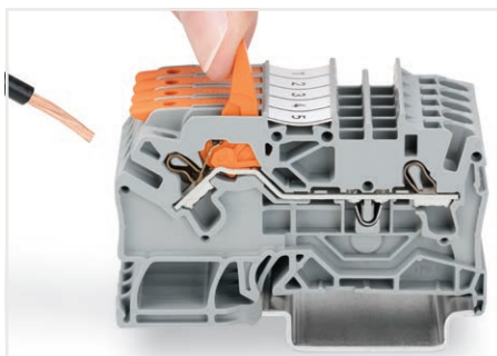
可とうより線 / より線： 操作レバーを上げて電線を挿入し、操作レバーを下げるだけで結線できます ※プッシュイン接続できない細い単線およびフェールル圧着線もレバー操作で結線可能です ※プッシュボタン操作側はP7を、ドライバ操作側はP8をご参照ください
