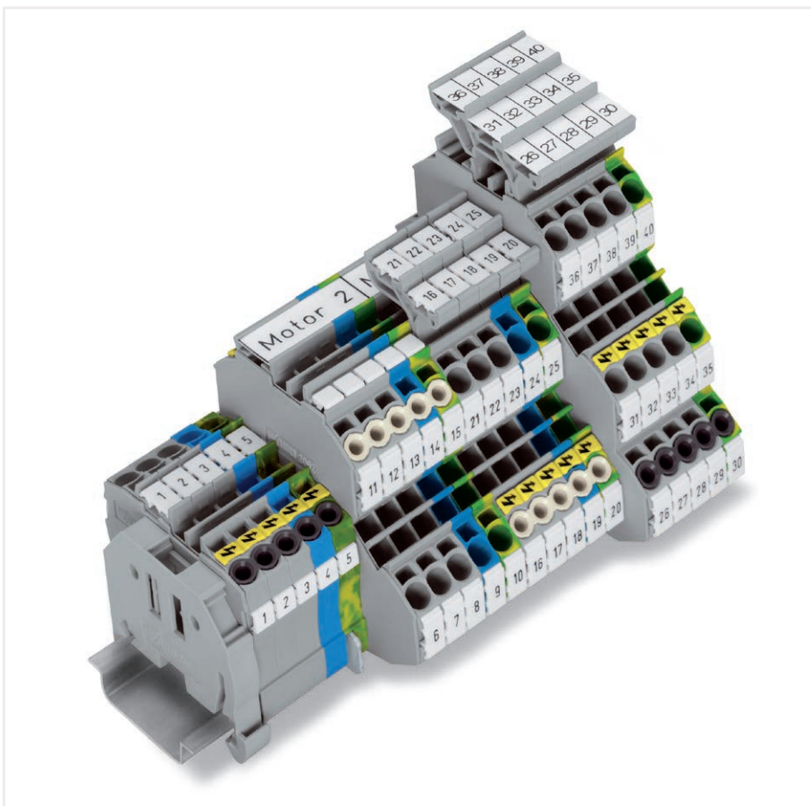
テストプラグアダプタを取り付けることで Ø 4 mm テストプラグまたはバナナプラグを使用した導通試験が可能です
