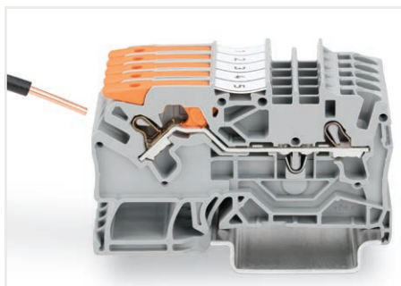
単線およびフェールル圧着線： 電線を差し込むだけのプッシュイン接続です
