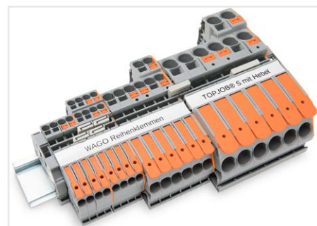
プッシュボタン操作 / ドライバ操作の端子台を組み合わせて、シリーズ共通のアクセサリを使用できます。
