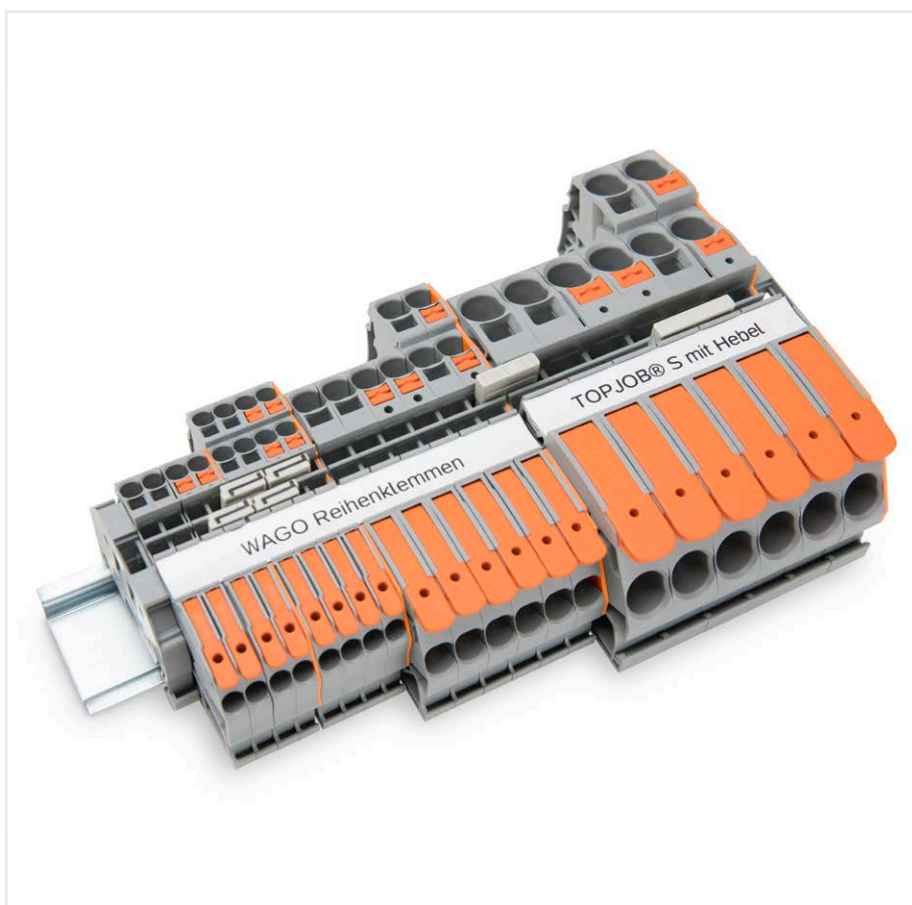
可とうより線 / より線： 操作レバーを上げて電線を挿入し、操作レバーを下げるだけで結線できます ※プッシュイン接続できない細い単線およびフェールル圧着線もレバー操作で結線可能です ※プッシュボタン操作側はP7を、ドライバ操作側はP8をご参照ください
