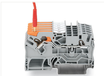
Ø 2 mm テストプラグを使用した試験 (最大 42 V)
